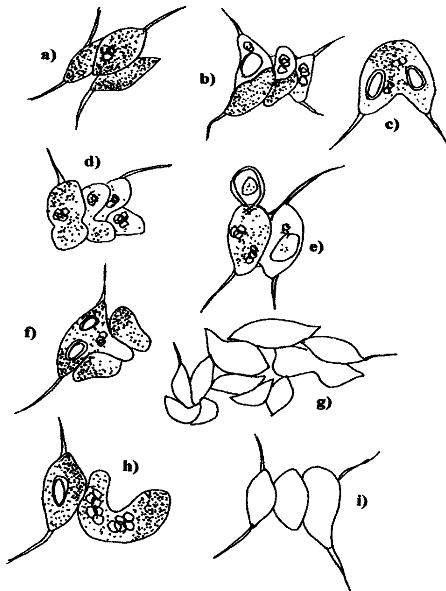
Obr. 1: Morfologie řasových cenobií Scenedesmus quadricauda
